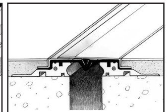
JDH 5.24 avec protection inox totale
